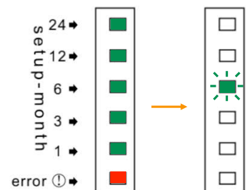
Abb. 7.2 Erstmaliger Betrieb
