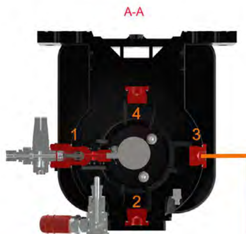
Abb. 14.1 Auslässe der Pumpe
