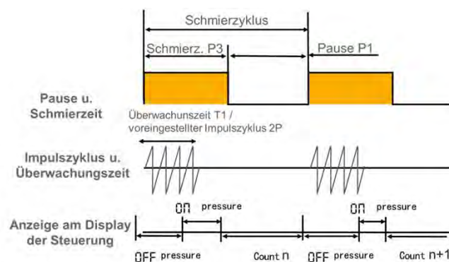
Abb. 25.3 T1 < 3P
