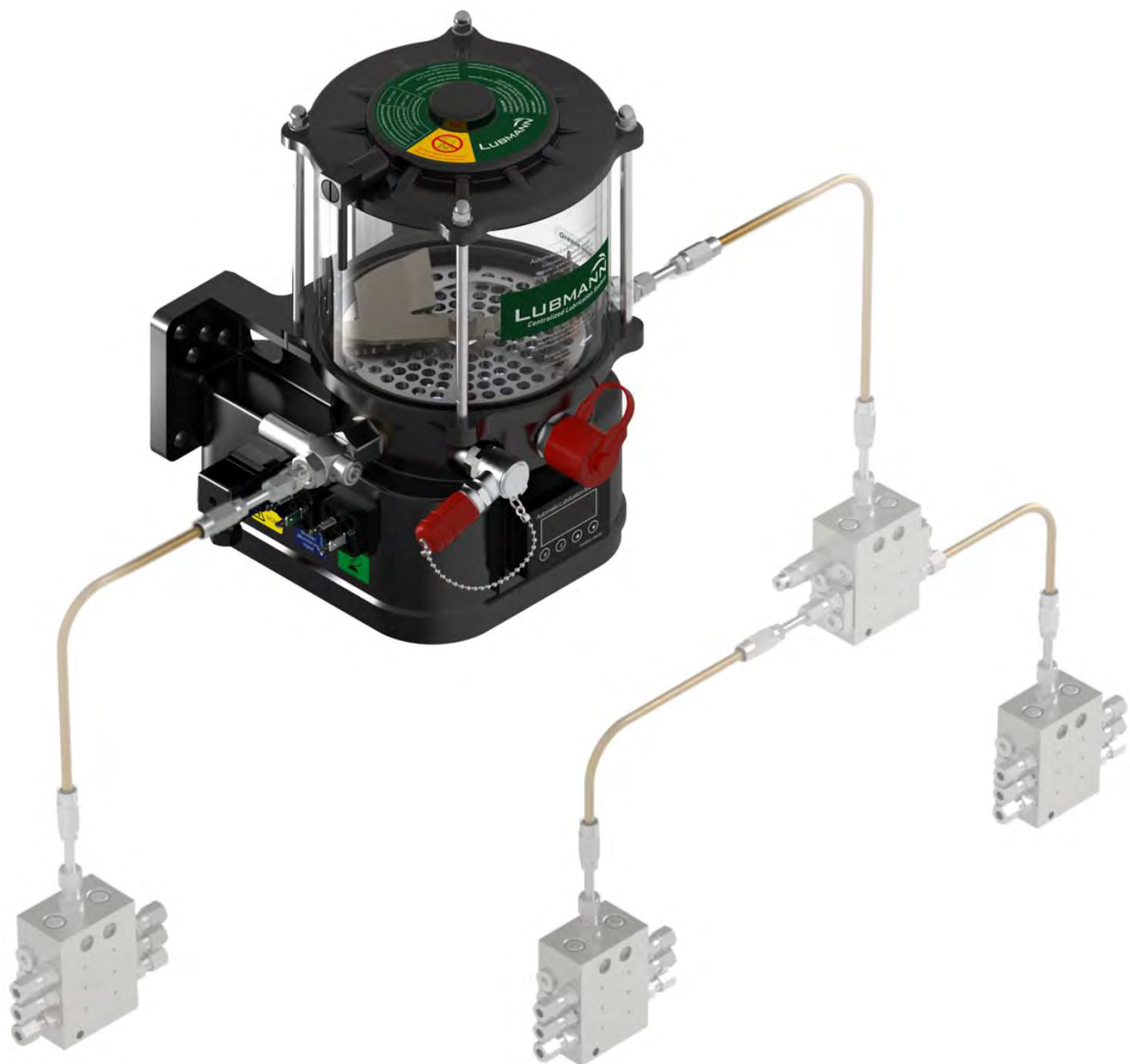
Abb. 11.1 Anlagenlayout für ALPB Progressivschmierpumpe + JPQ Progressivverteiler
