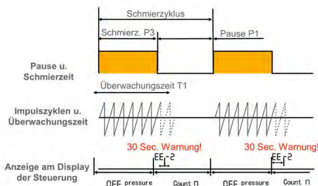
Abb. 25.4 T1 > 3P
