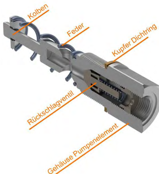
Abb. 14.2 Pumpenelement Aufbau
