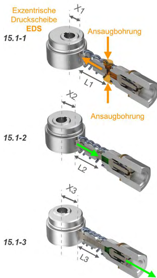
Abb. 15.1 Funktionsbeschreibung PE
