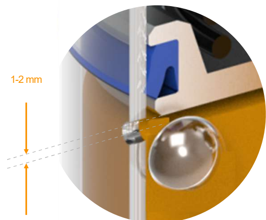
Abb. 5.2 Entlüftung des Behälters
