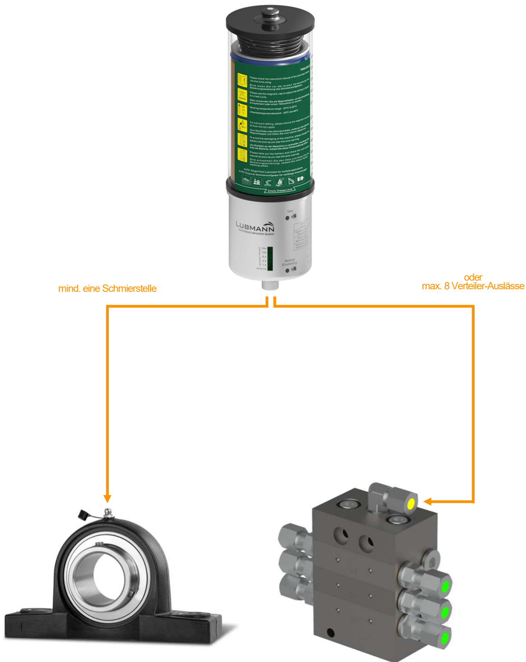
Abb. 3.1 Fettschmierpumpe-Einpunkt ALP01A verbunden mit Schmierstelle
