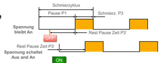
Abb. 3 Schmierzyklus ändert sich durch an u. abschalten während der Pausenzeit
