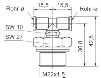
Anschlussverschraubung aus Kit-Zweiseitiger Bypass
