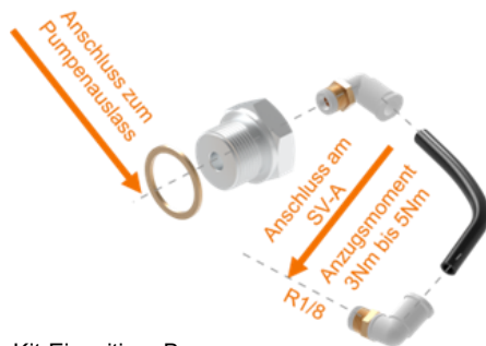
Kit-Einseitiger Bypass
