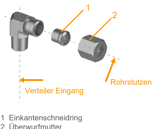
Abb. 11.1 Winkel Einschraubverschraubung
