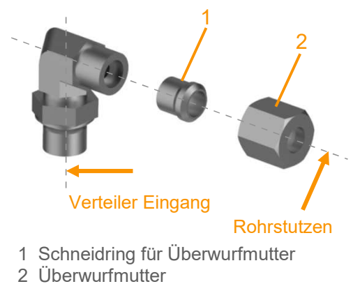
Abb. 12.2 Winkel-Einschraubverschraubung
