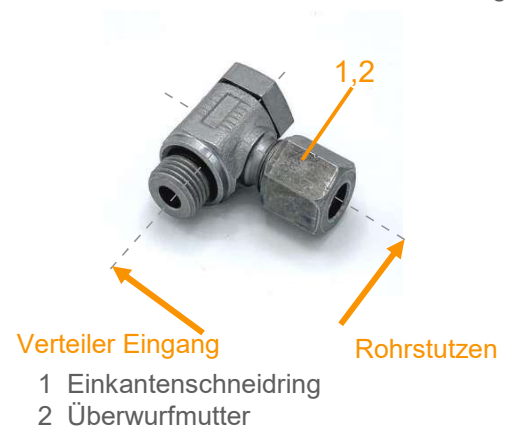
Abb. 12.2 Winkel-Einschraubverschraubung
