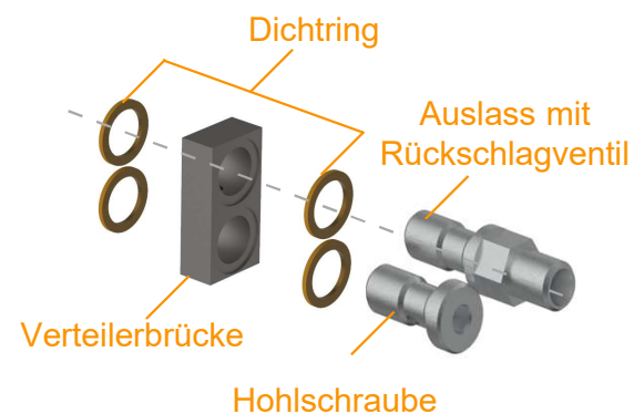
Abb. 18.2 Kit-Verteilerbrücke mit Auslass und Rückschlagventil
